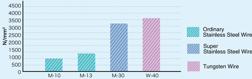
Comparison of tensile strength per mm 2
